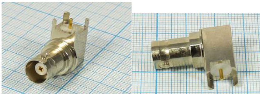
Разъем имеет позолоченный центральный контакт и хромированный корпус
