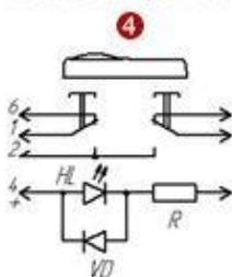
Электрическая схема коммутации
