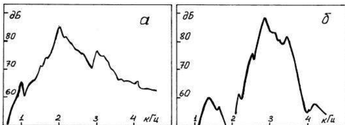
Рис.5. а) Частотная характеристика широкополосного звонка ПВА-1;
