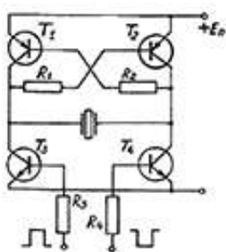
Рис.21. Мостовая схема оконечного устройства питаемая повышенным (десятки вольт) напряжением. Транзисторы: T1, T2 - КТ-502Г, КТ-973А, КТ-8147А T3, T4 - КТ-503Г, КТ-972А, КТ-8116А Резисторы R1 – R4 5 – 10 кОм.
