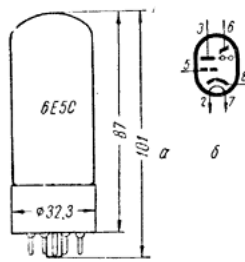
Рис. 204. Лампа 6E5C;
