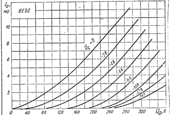
Рис. 207. Усредненные характеристики зависимости тока анода от напряжения на аноде при напряжении на кратере 250 в.
