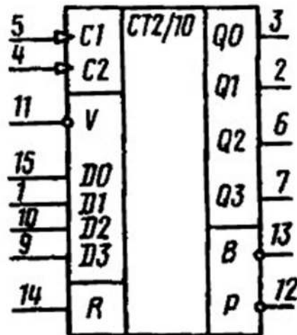
Условное графическое обозначение К555ИЕ6
