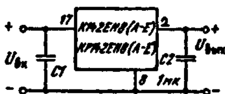
Типовая схема включения K142EH8 (A — E), KP142EH8 (A — E); C1 > 0,33 мкФ
