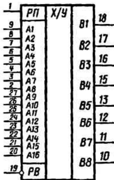
Условное графическое обозначение КР556РТ1
