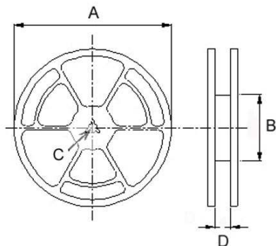
Reel Dimensions
