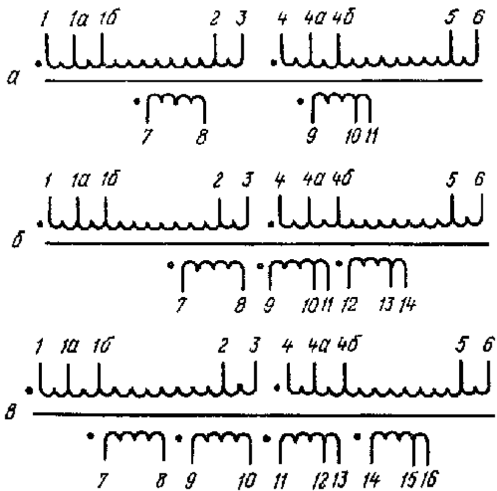
Рисунок 1. Электрические принципиальные схемы накаливающих трансформаторов ТН на броневых сердечниках ШЛ и ШЛМ на 50 Гц, 127/220 В: a - ТН1...ТН11, б - ТН12...ТН29, в - ТН30...ТН61
