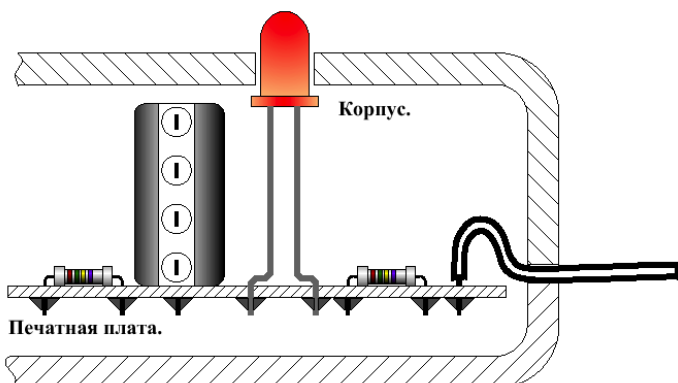
Рис.5 Установка светодиода на печатной плате
