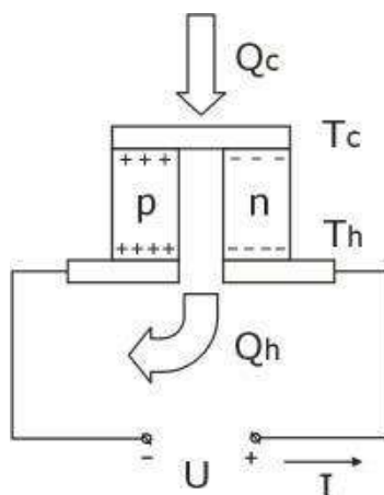
Рис.1 Схема действия эффекта Пельтье.
