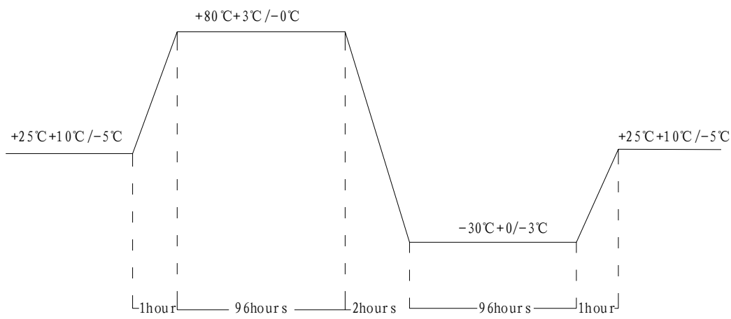
FIG1 TEMP. TEST
