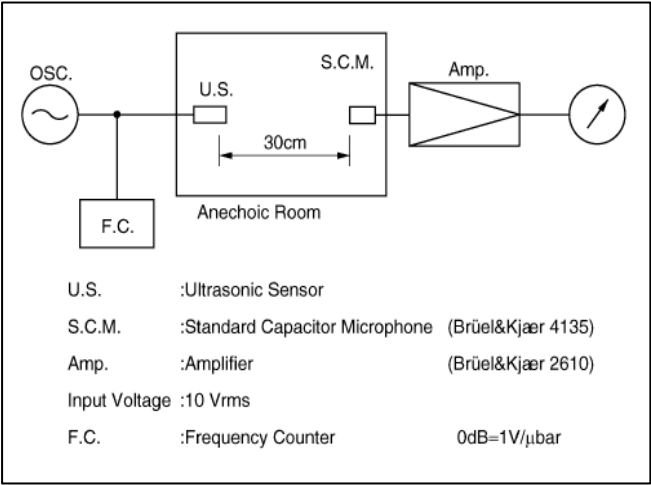
Transmitter发射
