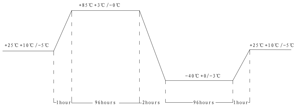
FIG1 TEMP. TEST
