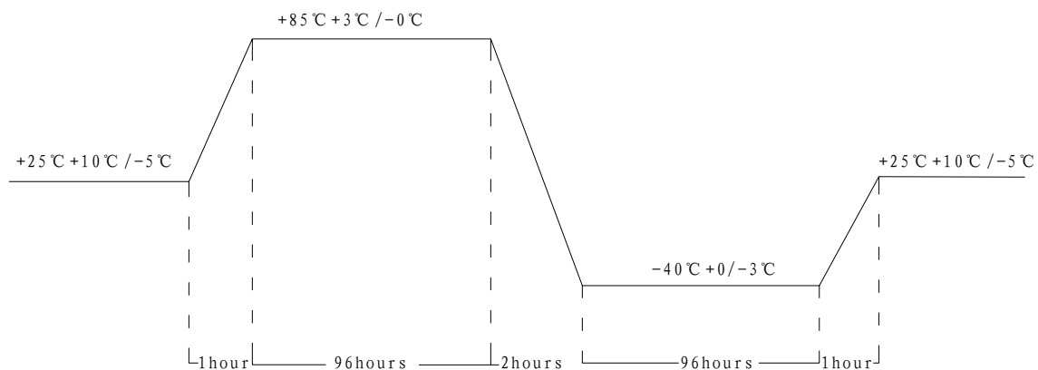
FIG1 TEMP. TEST
