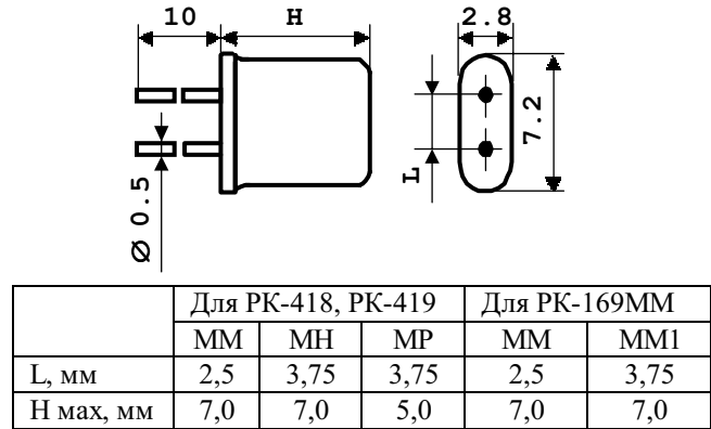
Рис 1. Корпус металлический типа ММ, ММ1, МН, МР
