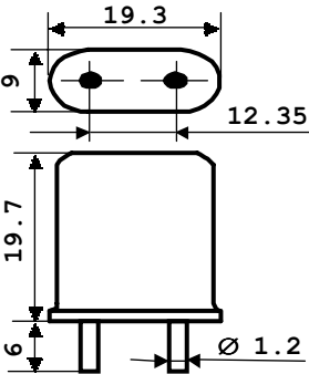
Рис.1 Корпус металлический типа Б
