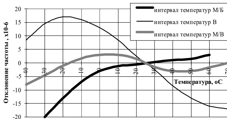
Рис 2. Типовые графики ТЧХ резонаторов РК418Т, РК419Т
