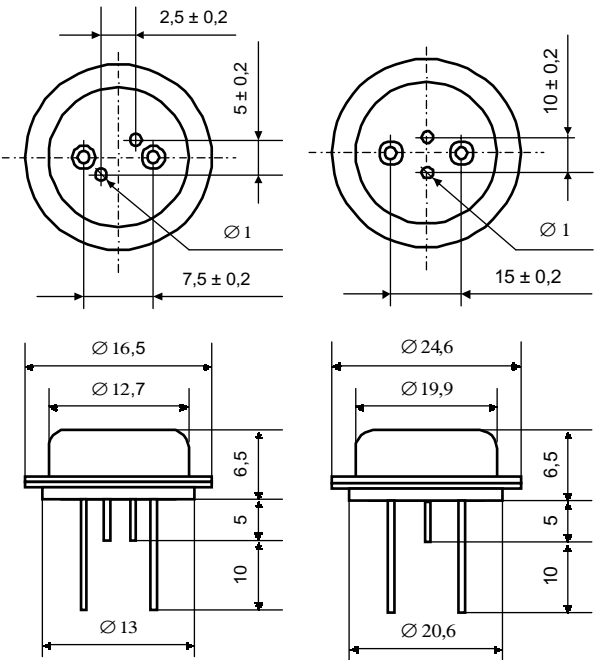
Рис.1 Корпус металлический типа ТА Рис.2 Корпус металлический типа ТБ
