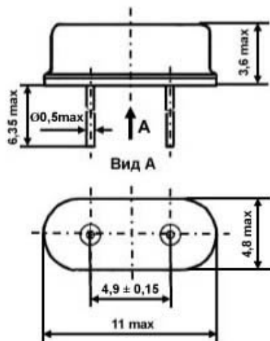
Габаритные, установочные и присоединительные размеры кварцевого резонатора РК415 для объемного монтажа
