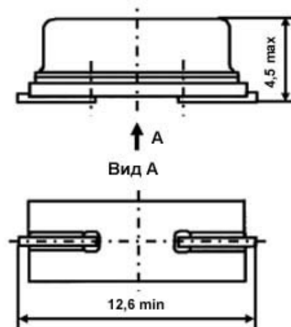
Габаритные, установочные и присоединительные размеры кварцевого резонатора РК415 (ТМП) для поверхностного монтажа
