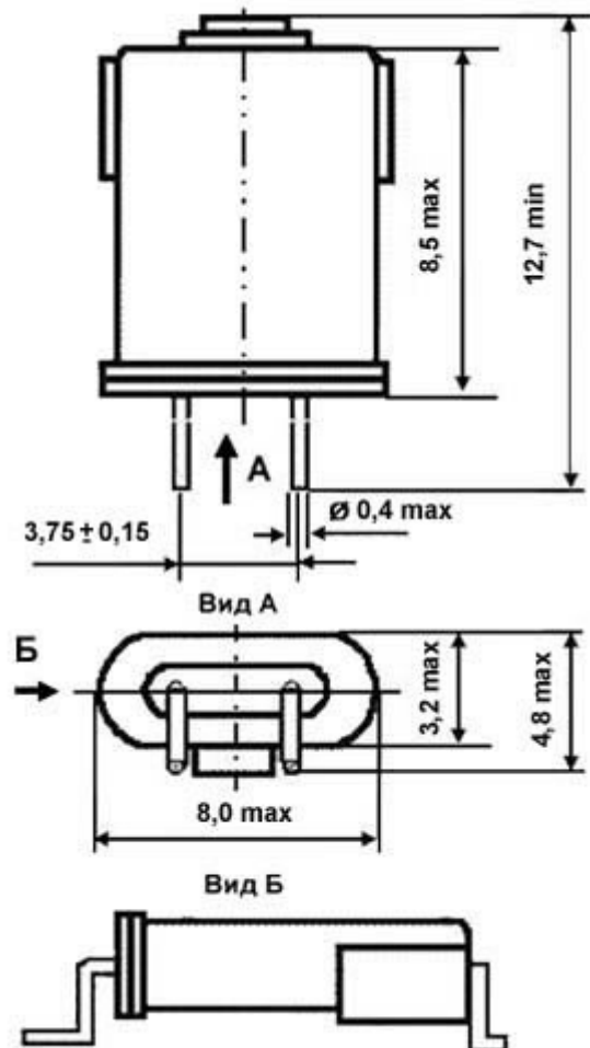
Габаритные, установочные и присоединительные размеры кварцевого резонатора РК454 (ТМП) для монтажа на поверхность
