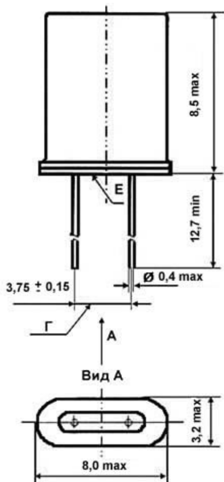
Габаритные, установочные и присоединительные размеры кварцевого резонатора РК454 для объемного монтажа
