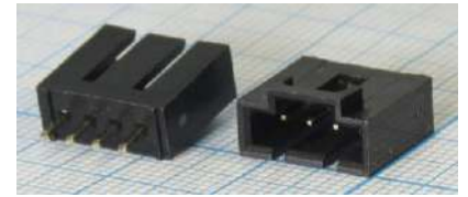
Штекер BL-4M
