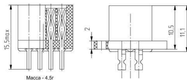
Рисунок 12 Розетка РГ1Н-1-7
