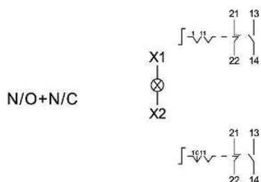
Электрическая схема коммутации
