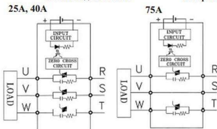
Схемы подключения
