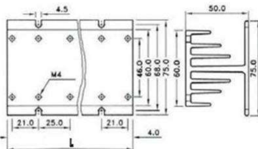
HS-□□□-H: Радиаторы для реле H-типа
