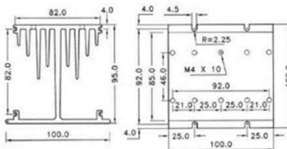
TSR-100 или HS-100: Радиаторы для трехфазных реле
