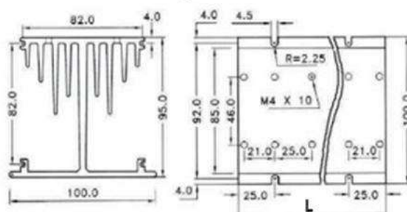
HS-□□□: Радиаторы для реле стандартного типа
