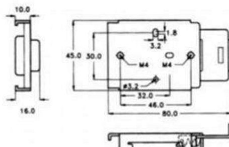
HS-BR-1: Радиаторы для установки на DIN-рейку
