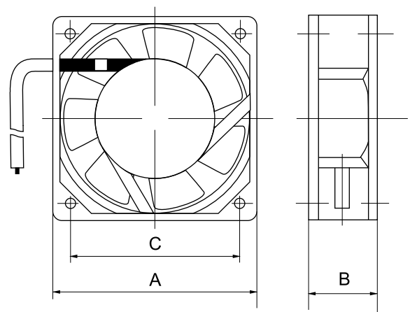
Чертеж №1
