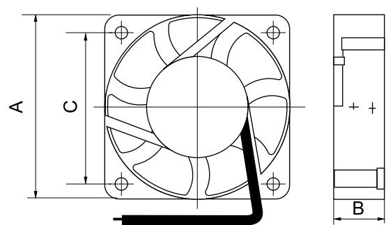
Чертеж №4
