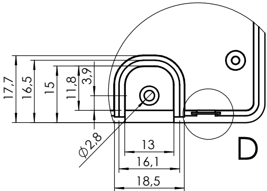
SZCZEGÓŁ C SKALA 1 : 1
