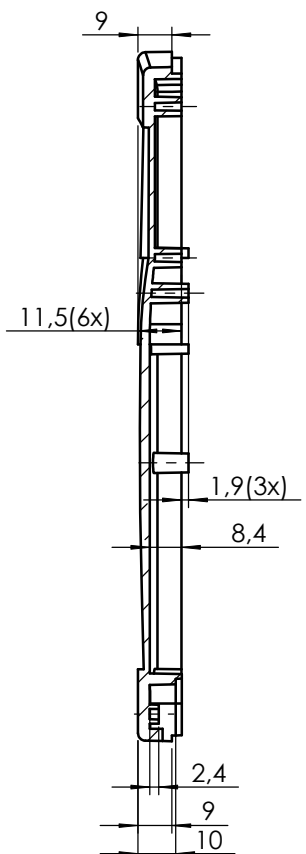
PRZEKRÓJ A-A
