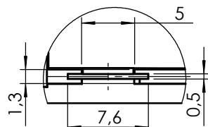
SZCZEGÓŁ D SKALA 2 : 1
