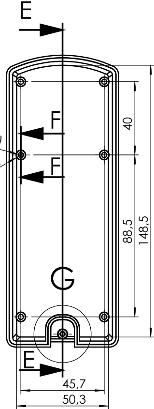
PRZEKRÓJ E-E
