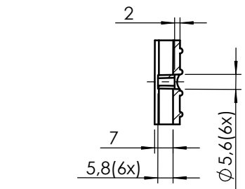
SZCZEGÓŁ G SKALA 1 : 1
