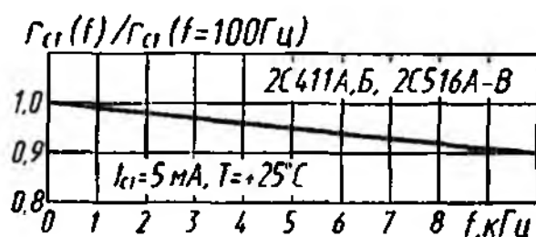
Зависимость дифференциального сопротивления от частоты
