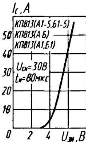
Зависимость тока стока от напряжения затвор—исток
