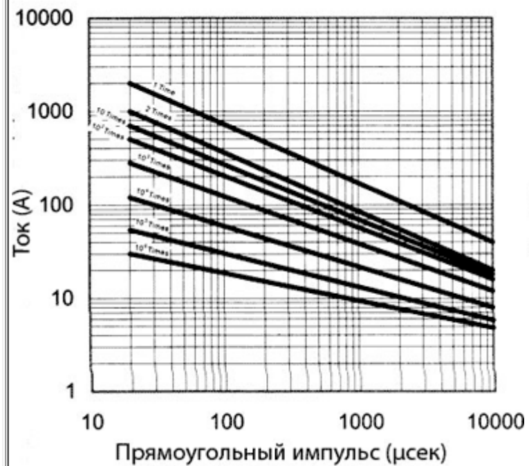
180LD20 - 680KD20
