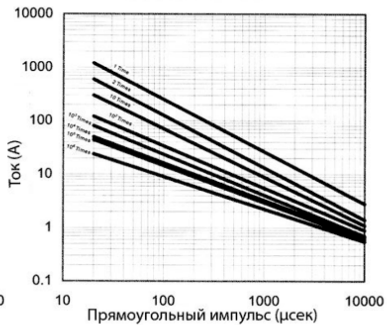
820KD07 - 821KD07
