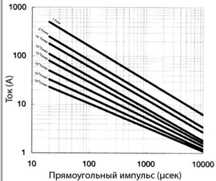
120MD10 - 680KD10
