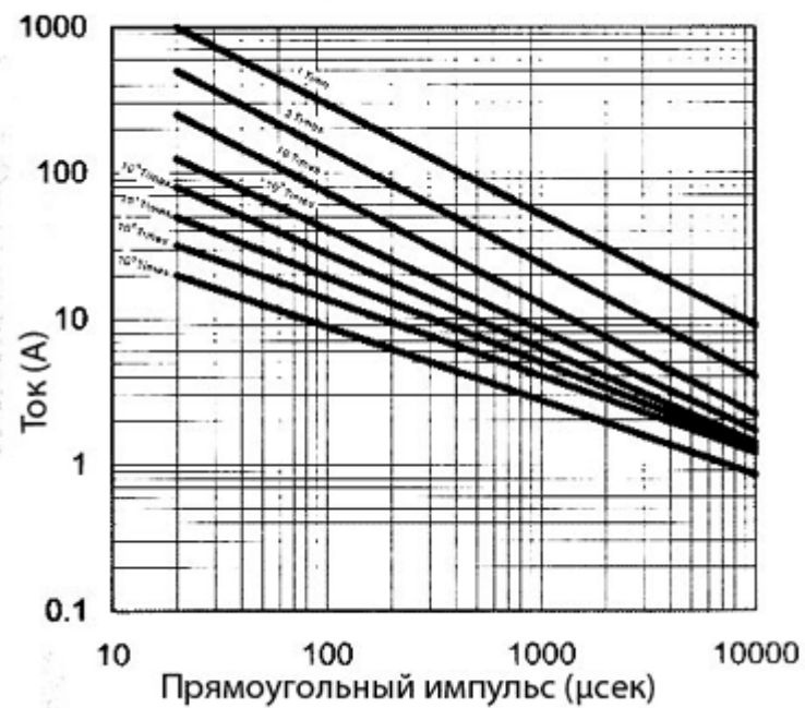
180LD10J ~ 680KD10J
