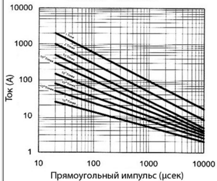
180LD14J - 680KD14J
