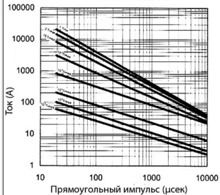
201KD25 - 182KD25
