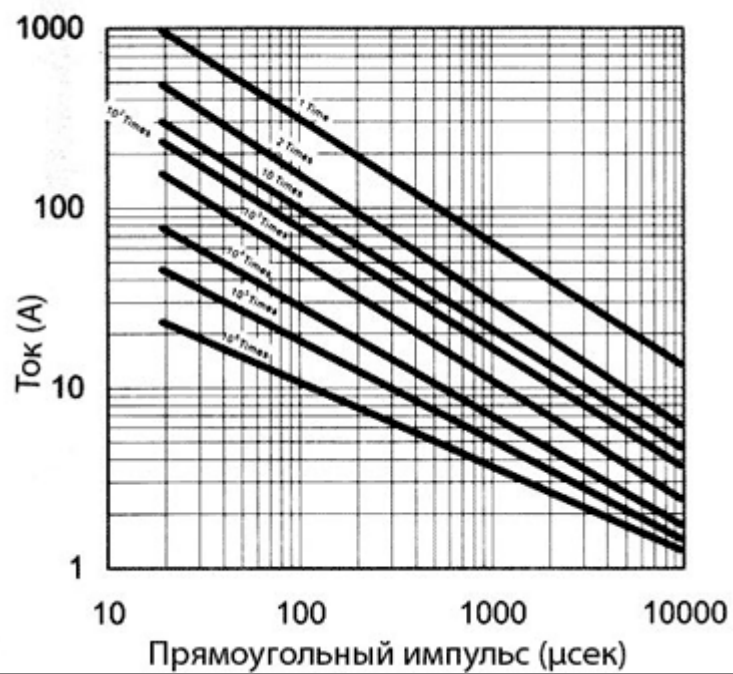
120MD14 - 680KD14
