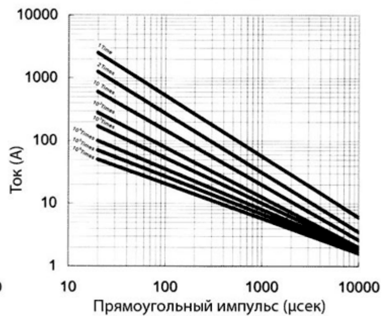
820KD10 - 112KD10
