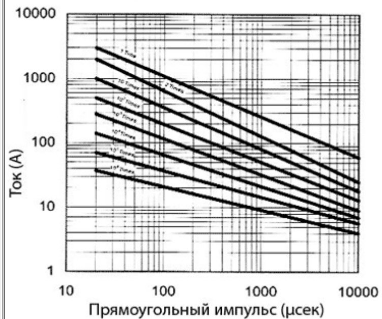
180LD20J - 680KD20J
