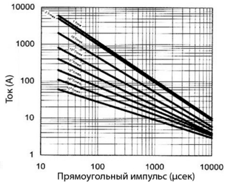
820KD14J - 182KD14J
