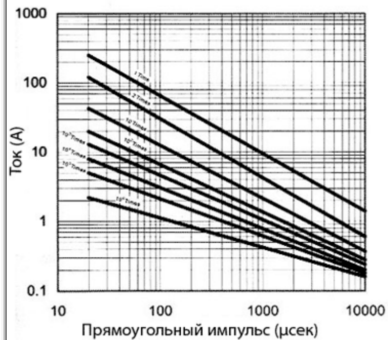
180LD05J - 680KD05J
