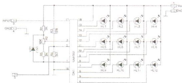
Рис.4 Схема электрическая принципиальная блока индикации «бегающая точка»
