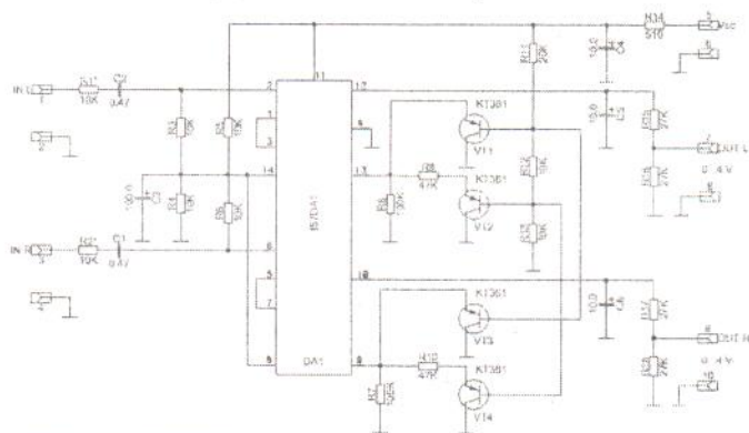
Рис.3 Схема электрическая принципиальная логарифмического детектора
