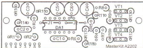
Рис.5 Схема расположения элементов на печатной плате логарифмического детектора
