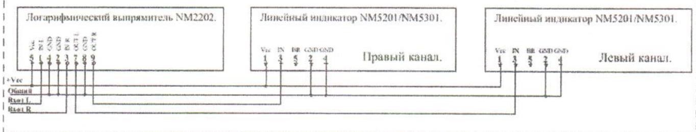
Рис.8 Схема соединений блоков
