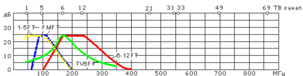
Типовая АЧХ
